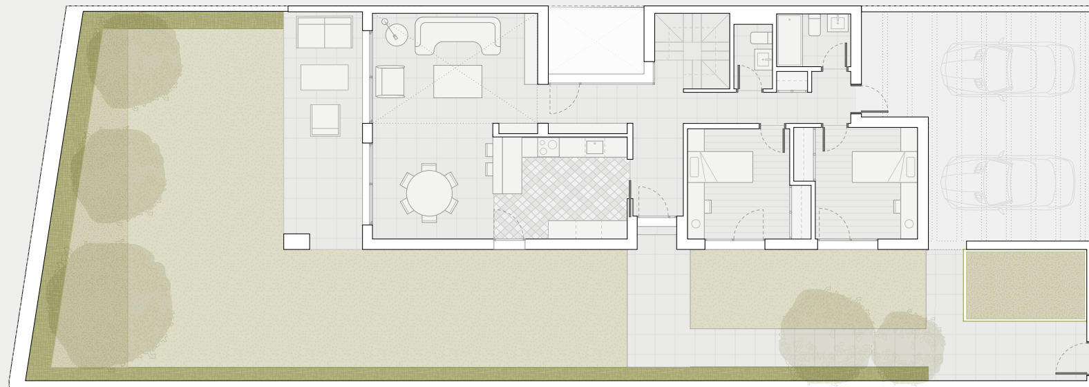
PLANTA BAJA
